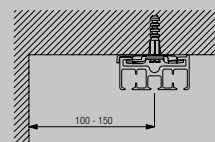
Deckenmontage mit Spanner 5320
