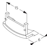
SG 10684 Osłona
